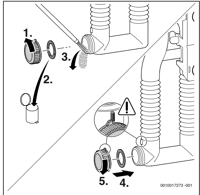
Joon. 53 Kondensaadisifooni puhastamine
