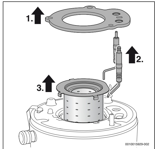
Joon. 46 Põleti väljavõtmine
