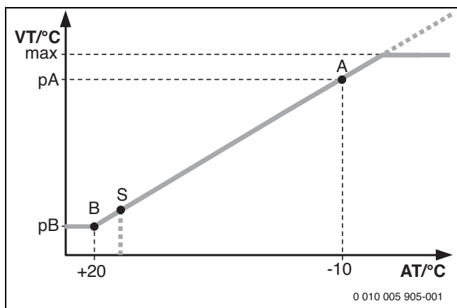
Joon. 74 Küttekarakteristik
