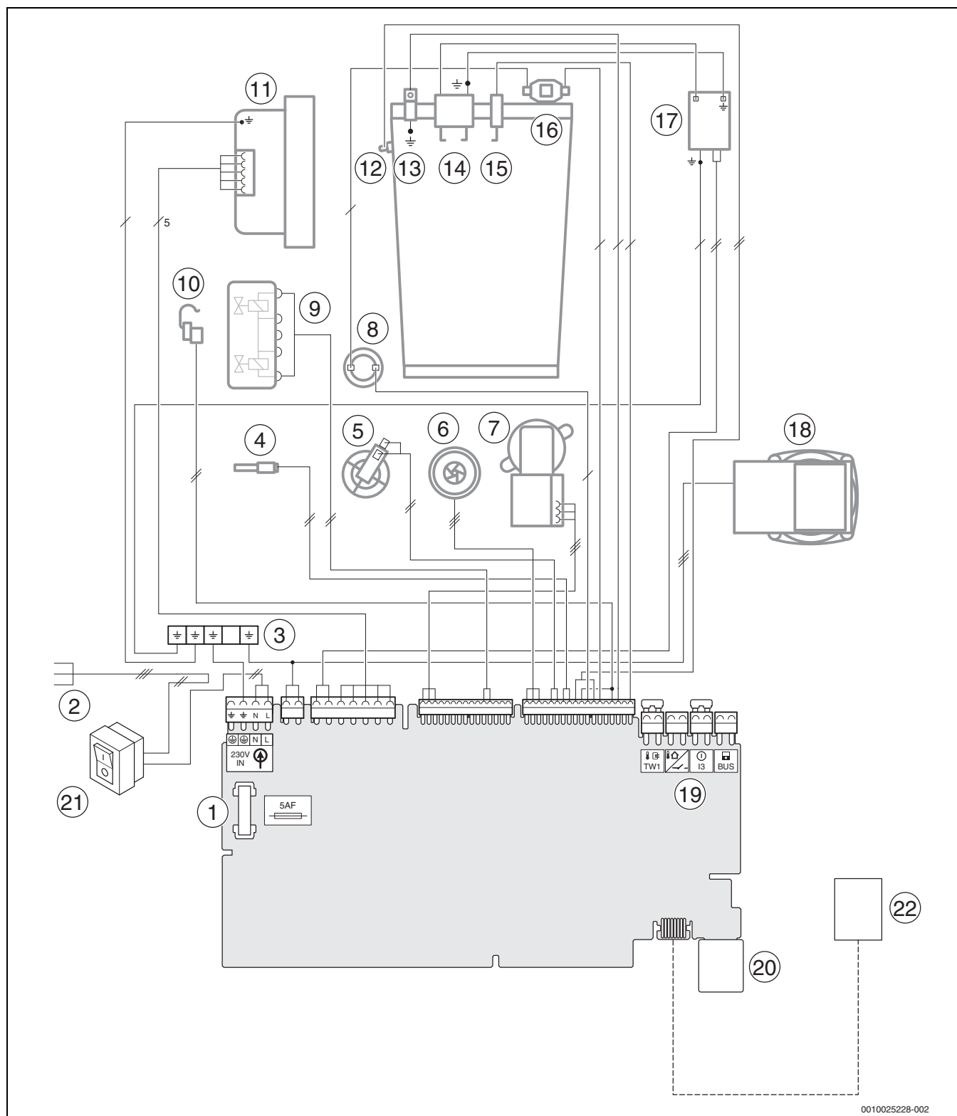
Joon. 73 Elektriühendused
