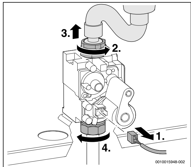
Joon. 61 Ühendada pistik lahti ja keerata kübarmutrid lahti.
