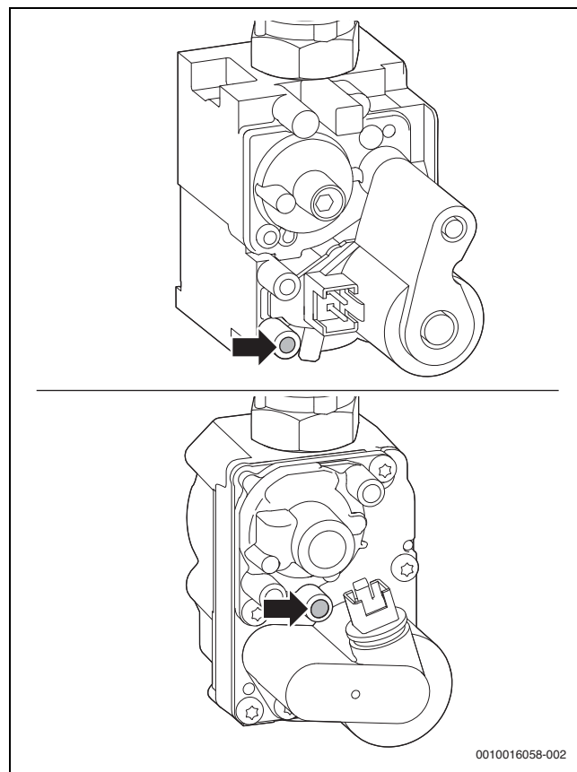
Joon. 40 Gaasivarustuse rõhu mõõtelitnik
