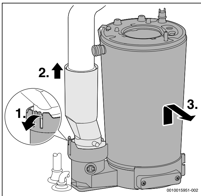
Joon. 67 Soojusvaheti eemaldamine
