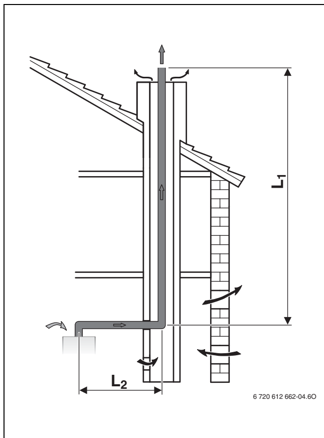
Joon. 8 Suitsutoru šahtis: B 23p
