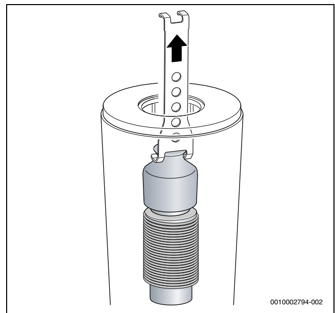
Joon. 47 Ülemise hajuti eemaldamine
