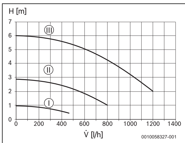
Joon. 36 Küttesüsteemi pumba karakteristik (püsiv rõhk)
