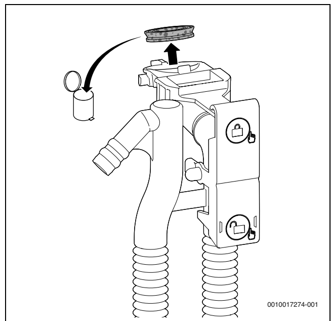
Joon. 54 Vahetage kondensaadisifooni ülaküljel olev tihend
