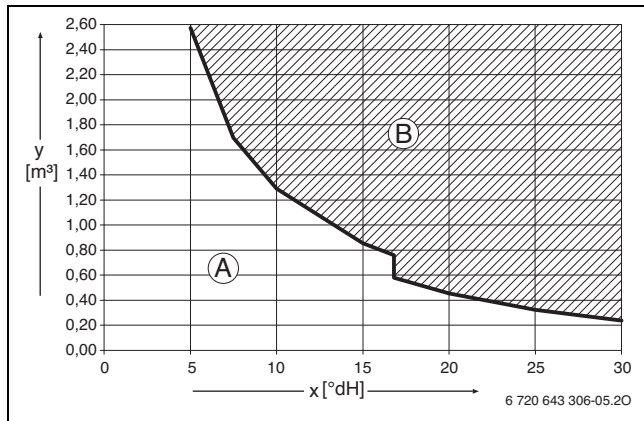
Joon. 21 Nõuded °dH täite- ja lisavee kohta &lt; 50 kW seadmetele
