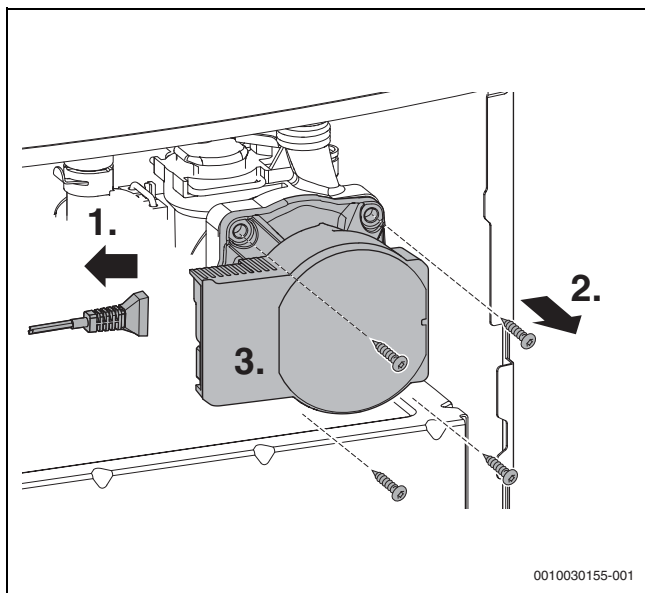
Joon. 63 Küttesüsteemi pumba eemaldamine
