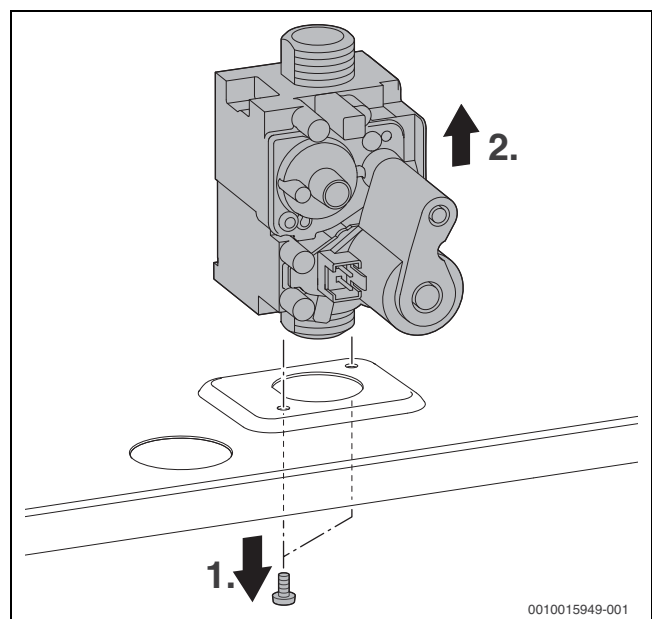
Joon. 62 Gaasiarmatuuri eemaldamine
