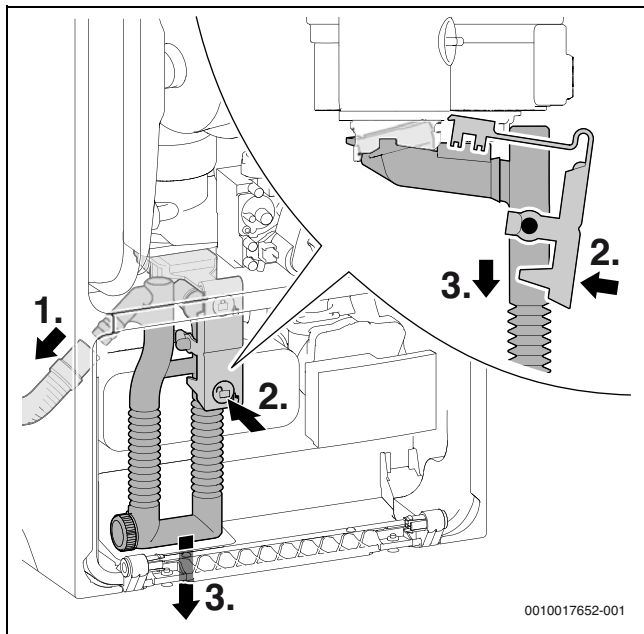
Joon. 52 Kondensaadisifooni eemaldamine
