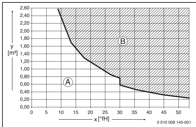
Joon. 22 Nõuded °fH täite- ja lisavee kohta &lt; 50 kW seadmetele
